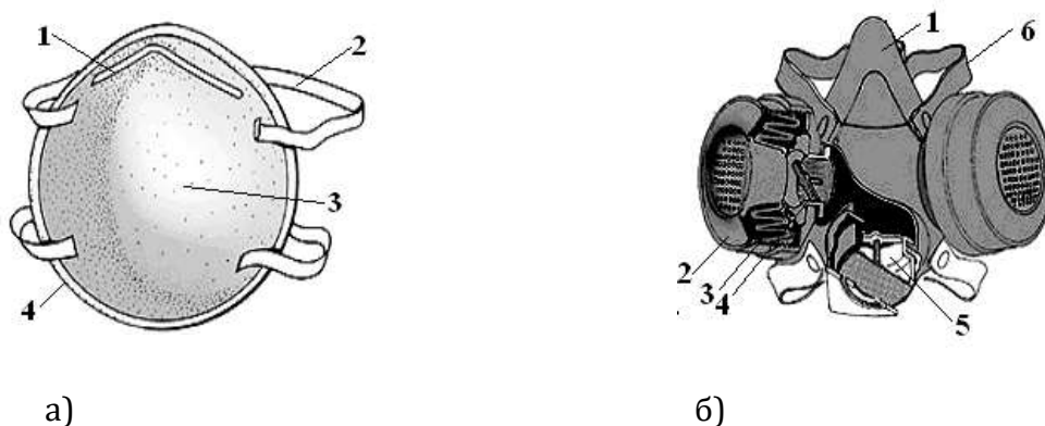
Рис. 1. Типи фільтрувальних ЗІЗОД: з фільтрувальною частиною (а): 1 - носовий затискач; 2 - наголів'я; 3 - фільтрувальна півмаска; 4 - обтюратор; з еластомірною півмаскою (б): 1 - півмаска з еластичного матеріалу; 2 - фільтрувальна коробка; 3 - фільтр; 4 - клапан вдиху; 5 - клапан видиху; 6 - наголів'я
