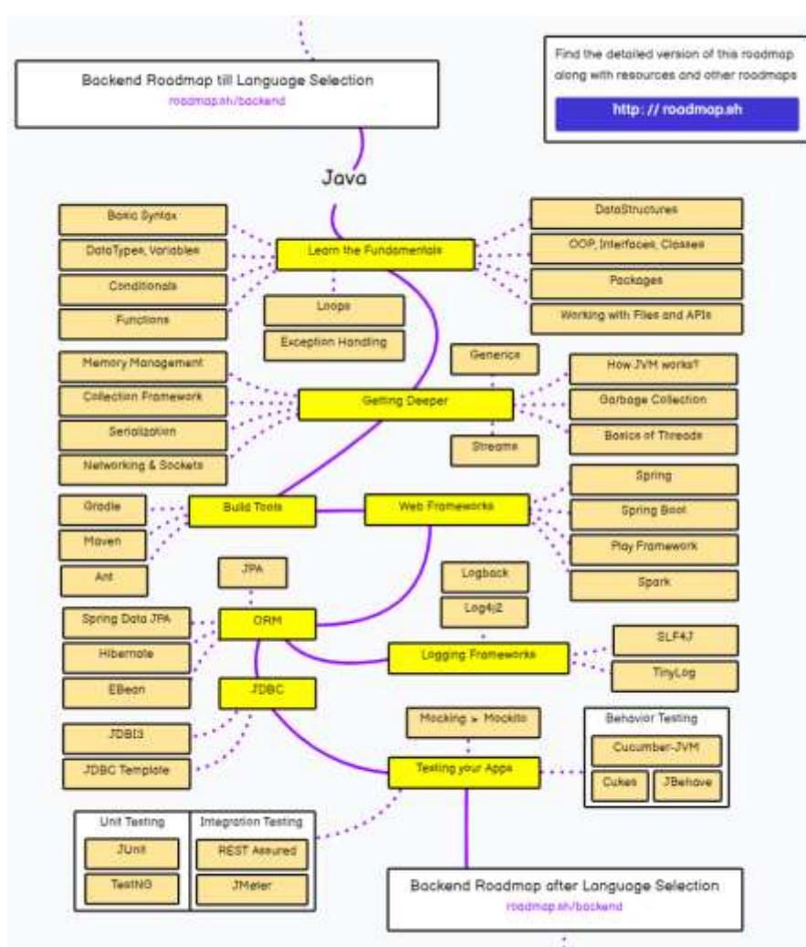
Рис. 1. Приклад побудови дорожньої карти для вивчення мови Java [2]
